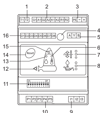
Рис. 14 Модуль IO 111
