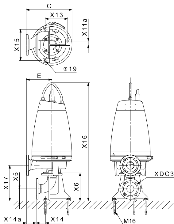
Рис. 11 SE1 Dry vertical
