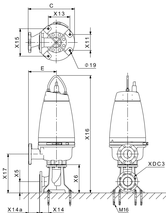
Рис. 13 SEV Dry vertical
