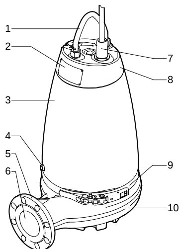
Рис. 1 Насос SE
