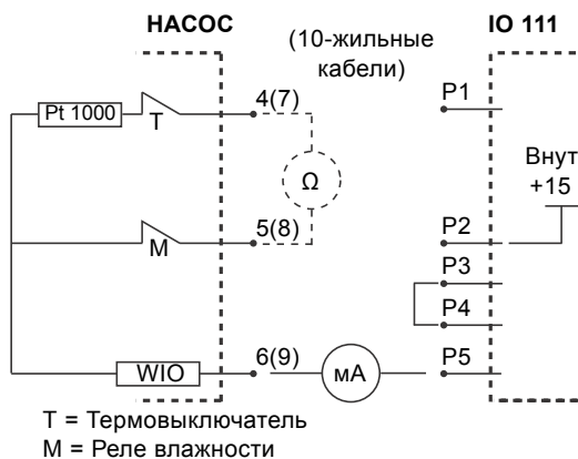
Рис. 24 Насосы SE1, SEV с Pt1000
