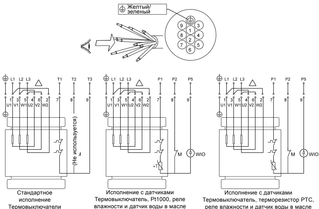
Рис. 11 Схема электрических соединений для 10-жильного кабеля, соединение треугольником (D)
