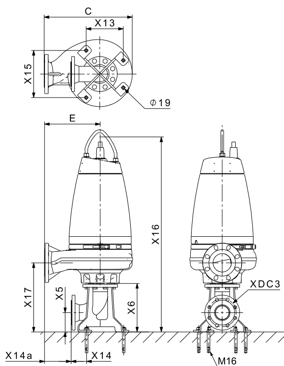
Рис. 12 SE1 Dry vertical
