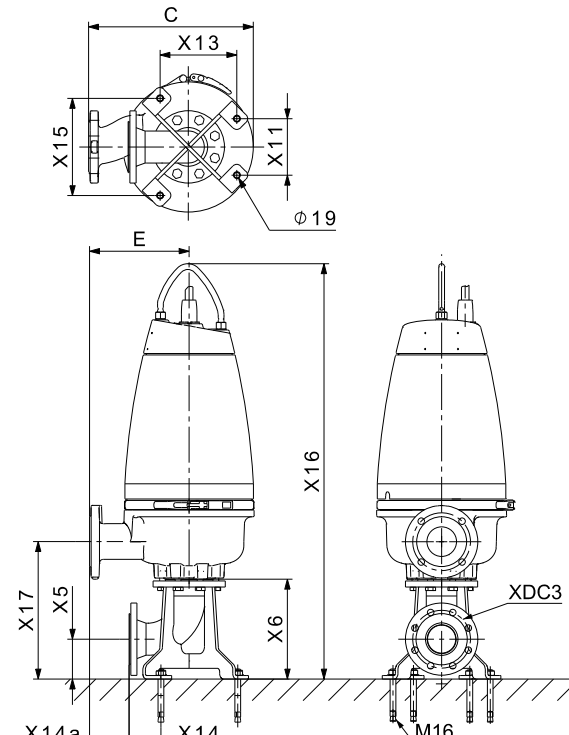
Рис. 14 SEV Dry vertical
